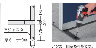
アンカー固定も可能です。
