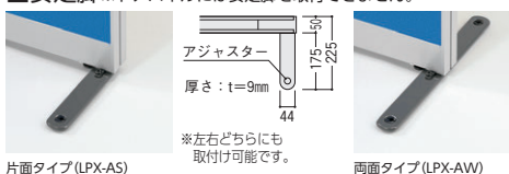
片面タイプ(LPX-AS) 両面タイプ(LPX-AW)
