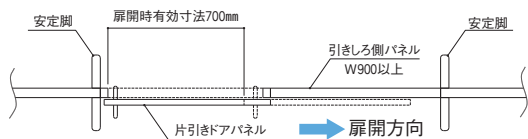
片引きドア取付例 (右引き扉)
