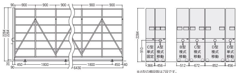
●7連式正面図
