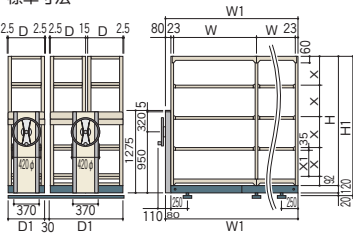
呼び寸法H2100×W1460×D300 天地6段
