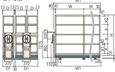
呼び寸法H2100×W1500×D471 天地6段
