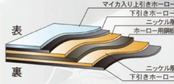
板面 断面図
