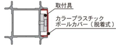
ポール断面図
