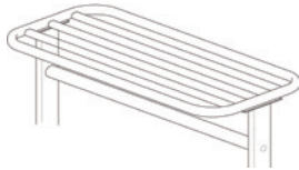
上棚詳細
